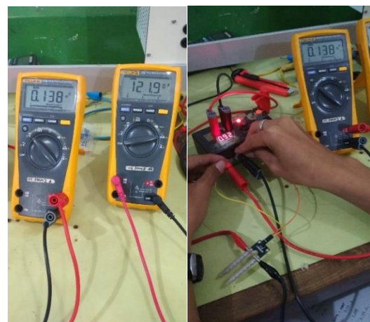
Gambar 13. Hubung singkat bagian 7 probe
